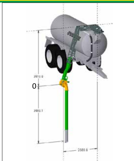
Rugzuikarm ingeklapt op de draaipunt boven vooraan op de tank (de waarden variëren naargelang van de gekozen configuratie)
