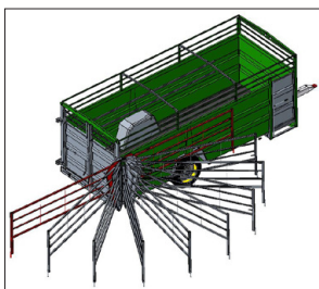
Posiciones de una barrera articulada
