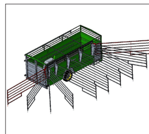
Posiciones de una barrera articulada en rieles
