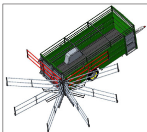
Posiciones de una barrera telescópica
