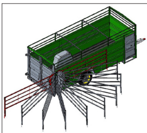
Position der schwenkbaren Gitter
