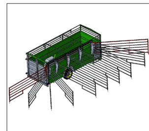
Position der schwenkbaren Gitter auf Führungsschienen
