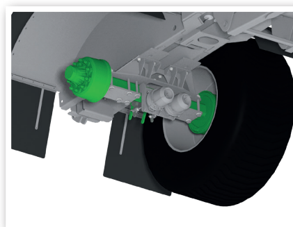
Przestawny układ jezdny
