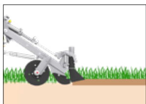
Injector cu patine conice și discuri de tăiere
