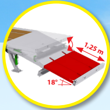
Telescopische laadbrug (1,25 m)
