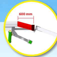
Geneigte Verlängerung bei gezogenen Modellen mit hydraulischen oder manuellen Rampen
