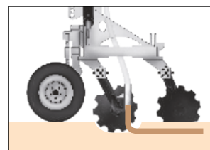
Культиваторный инжектор с дисками
