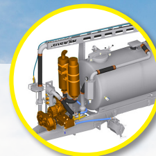
Промышленный насос производительностью 18 000 л/мин • Насос высокого давления 120 л/мин при 120 бар
