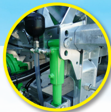
Suspensión hidráulica de la lanza
