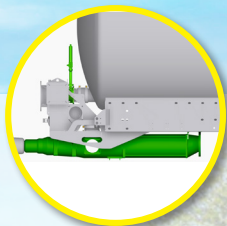
Pompe à colimaçon avec ramasse-pierres et pré-équipement pour Jumbo frontal
