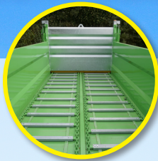
Doppelter Transportboden mit verschraubten Leisten und Schiffsketten Klasse 80
