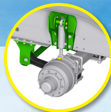
Hydro-Tandem: гидравлическая подвеска осей
