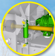
Hydraulische disselvering
