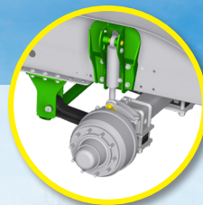
Hydro-Tandem : suspension hydraulique des essieux
