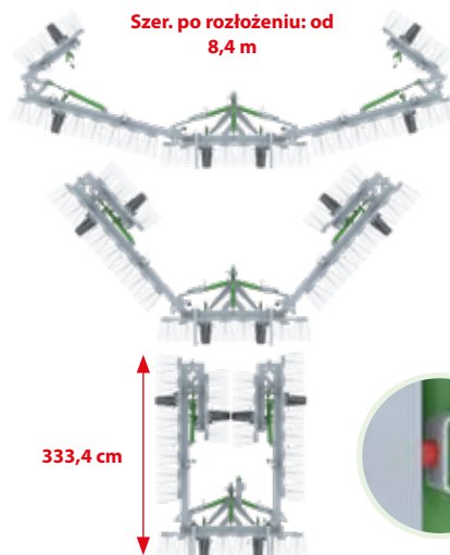
Podwójne składanie hydrauliczne z regulowanym odbojem z wygłuszającym Ertalonem do modeli o szerokości roboczej od 8,4 m.
