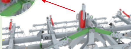
Variflex: bezstopniowa regulacja nacisku zębów ustawianych hydraulicznie za pomocą większej liczby siłowników kompensacyjnych i jednego lub dwóch siłowników centralnych z podziałką .
