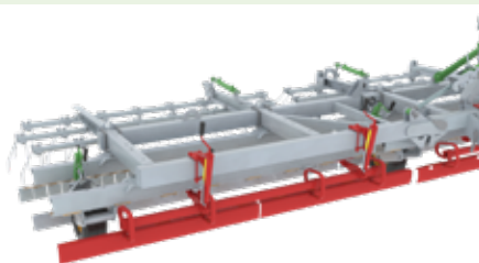
Niezależne listwy niwelujące o różnej szerokości (90 - 130 cm) zależnie od modelu, umieszczone przed kołami, by równać podłoże.
