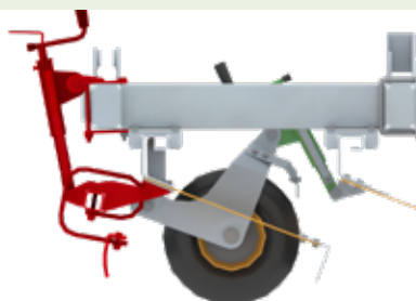
Regulacja wysokości listwy niwelujących za pomocą korby z podziałką i strzałką wskazującą.
